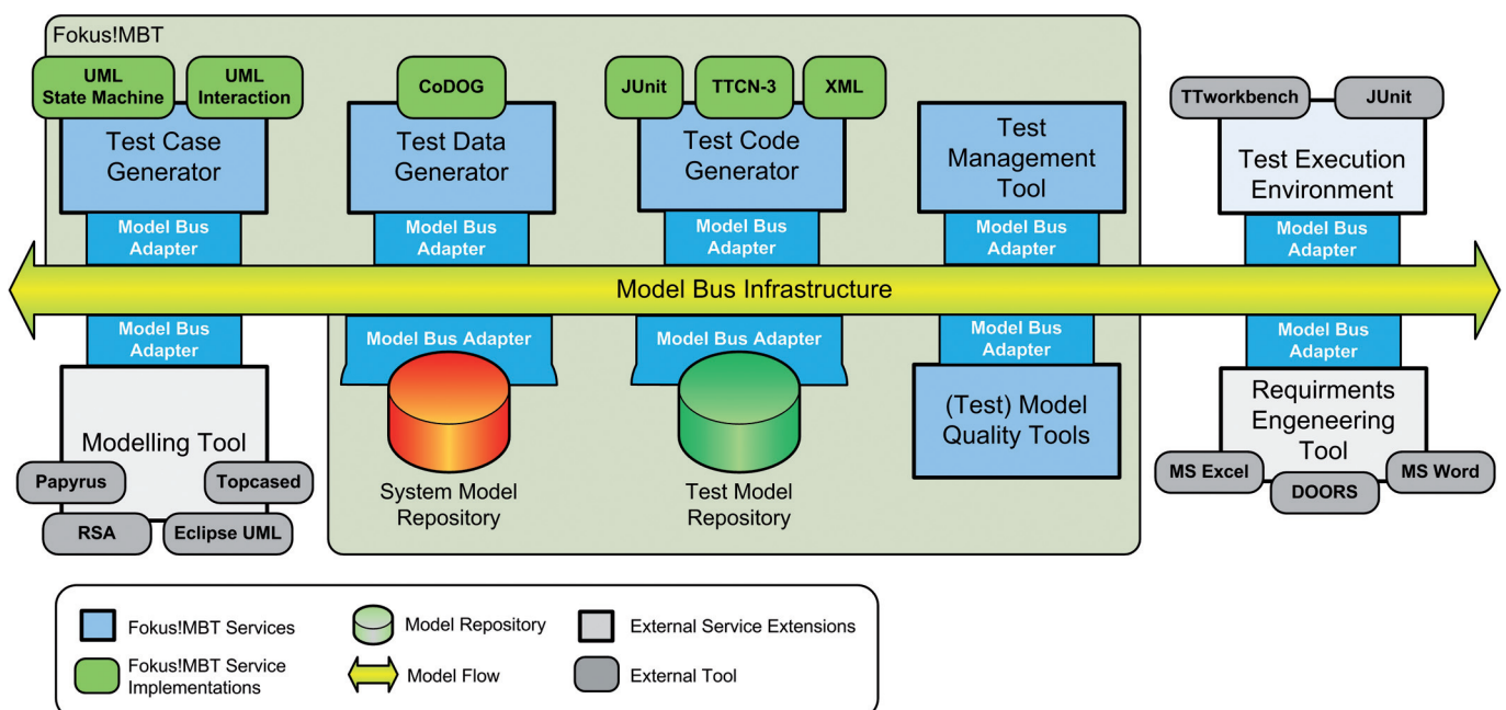
Abbildung 3: Architektur der Fokus!MBT-Werkzeugkette
