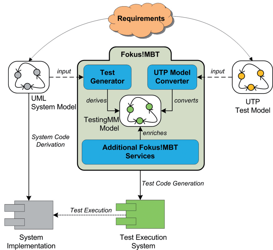
Abbildung 4: Fokus!MBT im Kontext manueller und automatisierter Ableitung des Testmodells
