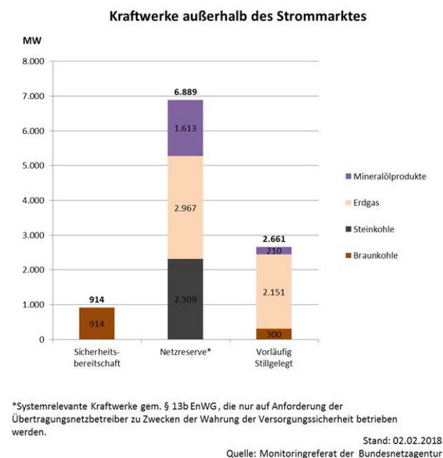
Abbildung 19: Kraftwerkliste der BNetzA 2018 [100].
